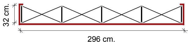
ESQUEMA SUPERIOR
